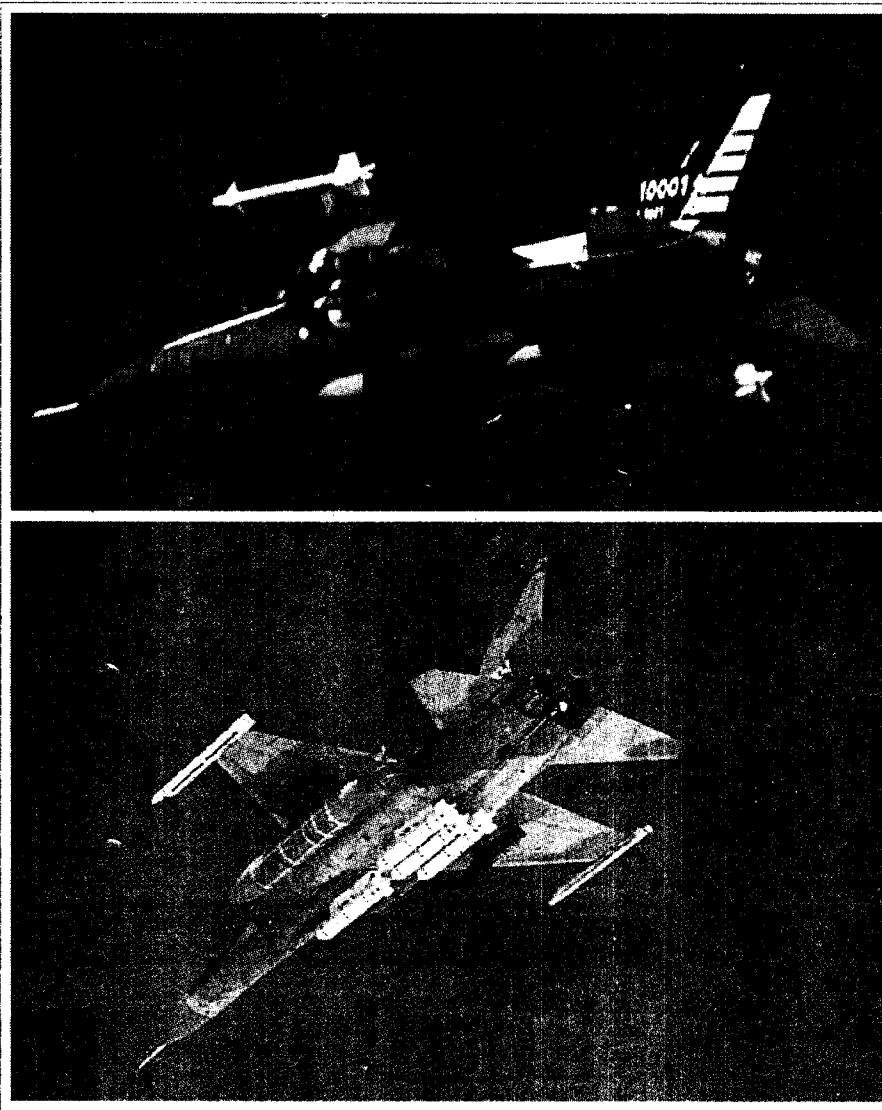
性過通已並，能性地對空的異優備具選，外能性戰作空對空除機戰號國經 IDF 為線中，彈飛空對空程短型一劍天用衛自掛梢翼機型原號一為圖上。估評試測能。彈炸速減磅百五枚六掛下翼，箱油副命加五七二束集枚四共線中腹機，式方載掛地對空的稱對不種一另試測機型原號四為圖下和力阻在證驗以，置空側右，箱油副命加五七二具一有邊左僅下翼右左但，彈炸。體軟系統控飛傳線和性定穩行飛，下變改心重將程航但，異小同 IDF 與型外，「台載制反合聯」的政研礎基為 IDF 以來未。務任「制反限有」行執，「器武制反」地對空院科中合配，伸延度速允德盧/文 供提司公翔漢/圖
