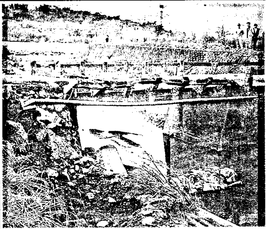
！下脚在就能可，橋危 候氣、舊老為因梁橋分部，梁橋損受座二廿百三有區地灣台布公天昨部通交 蓮花為園，心驚目慌人令，流車大龐來往有仍但，重慶沉情損受，刷沖川河及 供提部通交／圖 六見聞新 橋湖東
