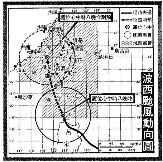
波西颶風動向圖
