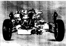
圖為全副裝配的明銳轎車底盤
