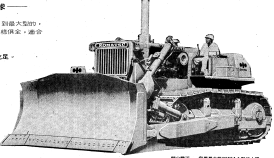
最大型推土機——D355A-1型推土機 (45.5噸、430HP、發動機44kg/cm²)
