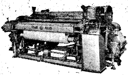
KRC-104 高速輪盤式換管自動織布機
