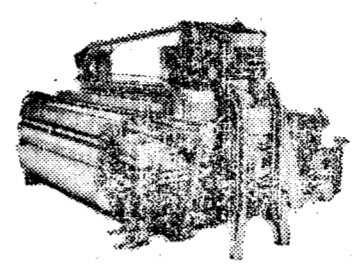
L-2 織機
