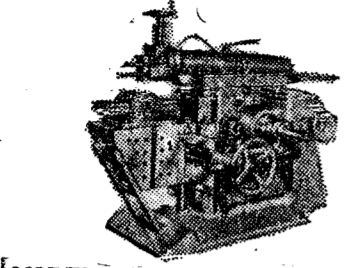
MODEL-600 24" 強力高速牛頭刨床
