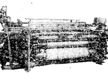
KSC-5 單面四梭格子織機
