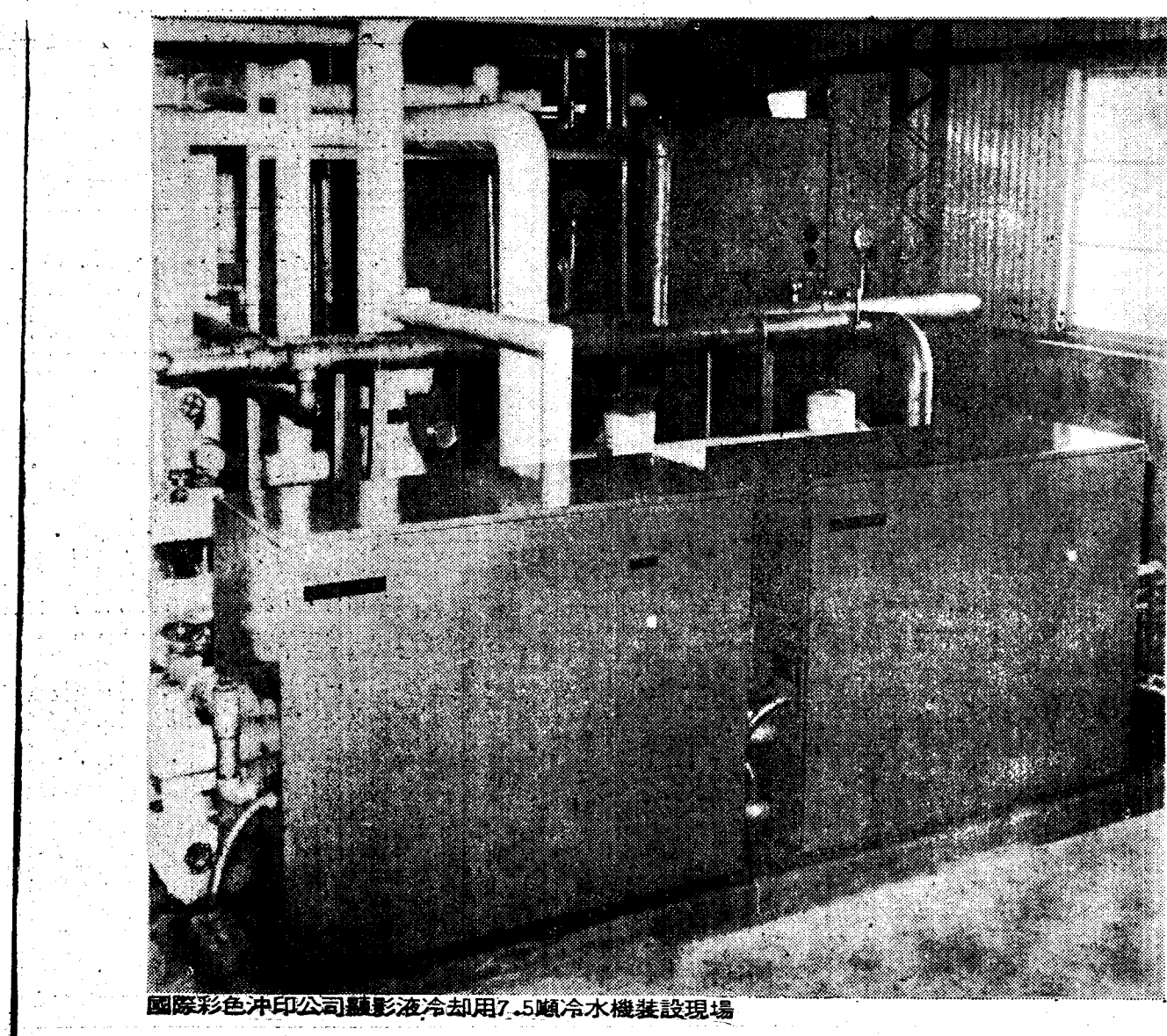
國際彩色沖印公司顯影液冷卻用7.5噸冷水機裝設現場
