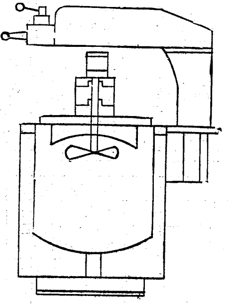
滴注式氣體滲炭爐
