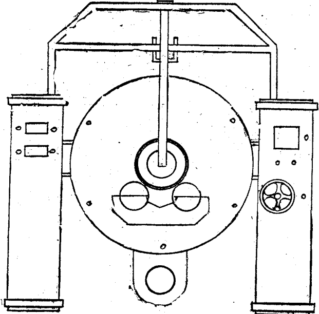
迴轉式氣體滲炭爐
