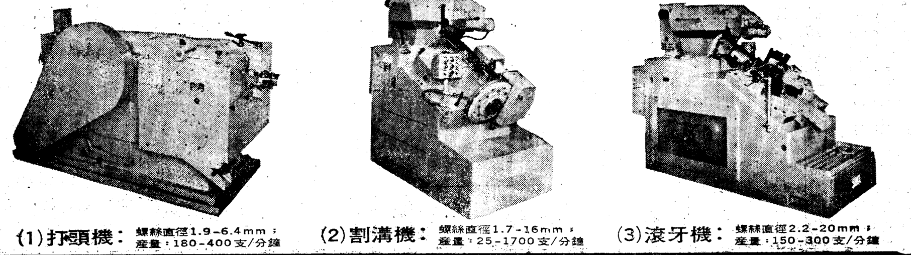
(1)打頭機：螺絲直徑1.9-6.4mm；產量：180-400支/分鐘 (2)割溝機：螺絲直徑1.7-16mm；產量：25-1700支/分鐘 (3)滾牙機：螺絲直徑2.2-20mm；產量：150-300支/分鐘
