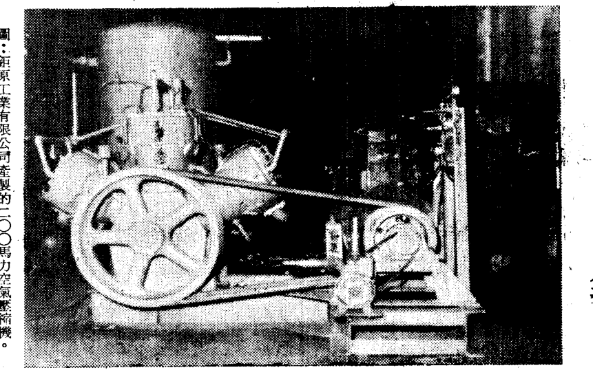
圖：永祥織造公司所製之20馬力空氣壓縮機。
