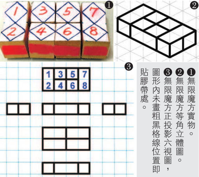
無線魔方零件圖的繪製及零件組合加工圖
