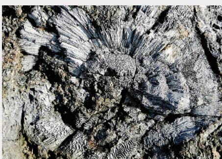
▲碳酸鈣膠結、重新結晶後形成石灰岩，岩石裡隱約可見珊瑚礁的形體。
