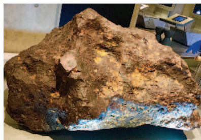
▲隕石是流星掉落地面的殘體。(展示於日本東京科博館)
