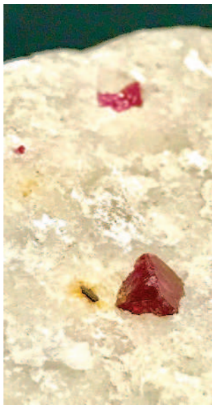
▲紅寶石是地球上珍稀的礦物。
