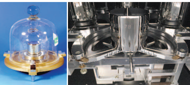
▲78號鉑鈱原器（左），放置於質量比較儀內（右）。
