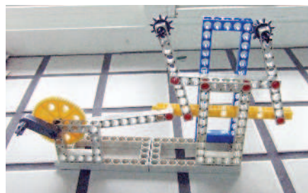
▲積木機關「週期運動」。
